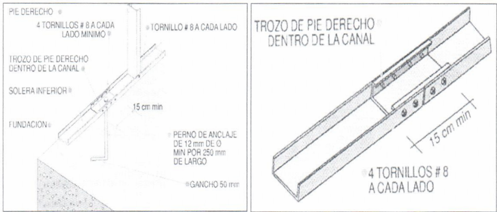
Fijación a Sobrecimientos
