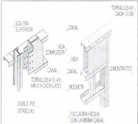
Estructuración dinteles de vanos
