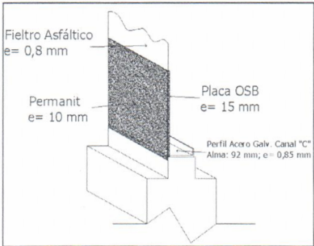
Estructuración revestimiento exterior de muros perimetrales
