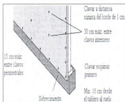
Fijación de placa OSB a estructura Metalcon
